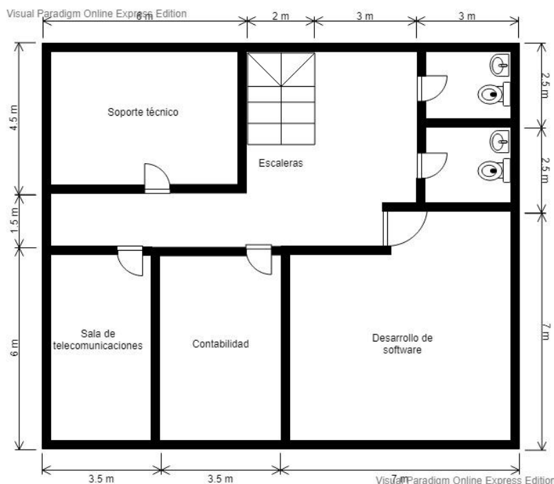
Figura 2. Segundo nivel. Nuevas instalaciones empresa Innova Soft.
