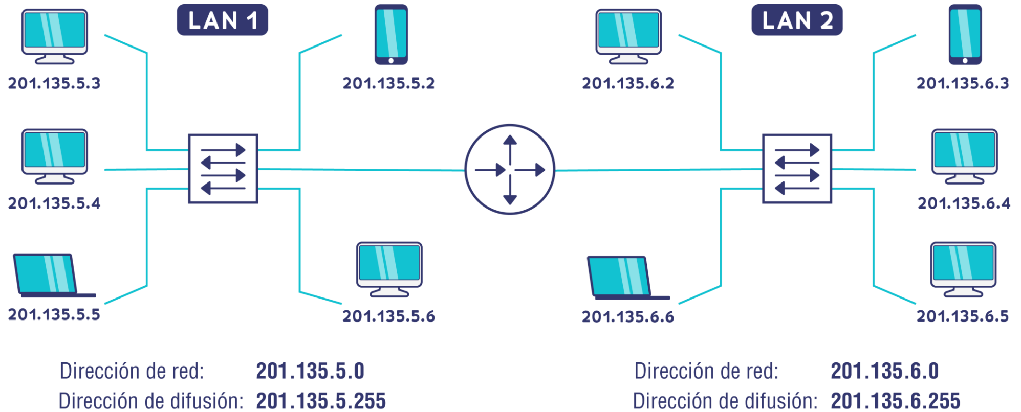
Figura 3. Conexión de dos LAN.
